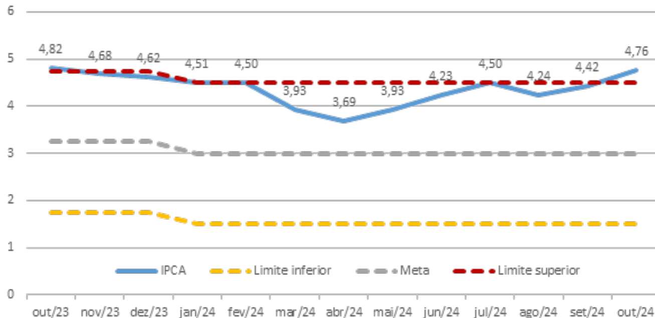
Gráfico 5 - Brasil: Variação (%) Acumulada do IPCA em 12 meses - out/2023 a out/2024
